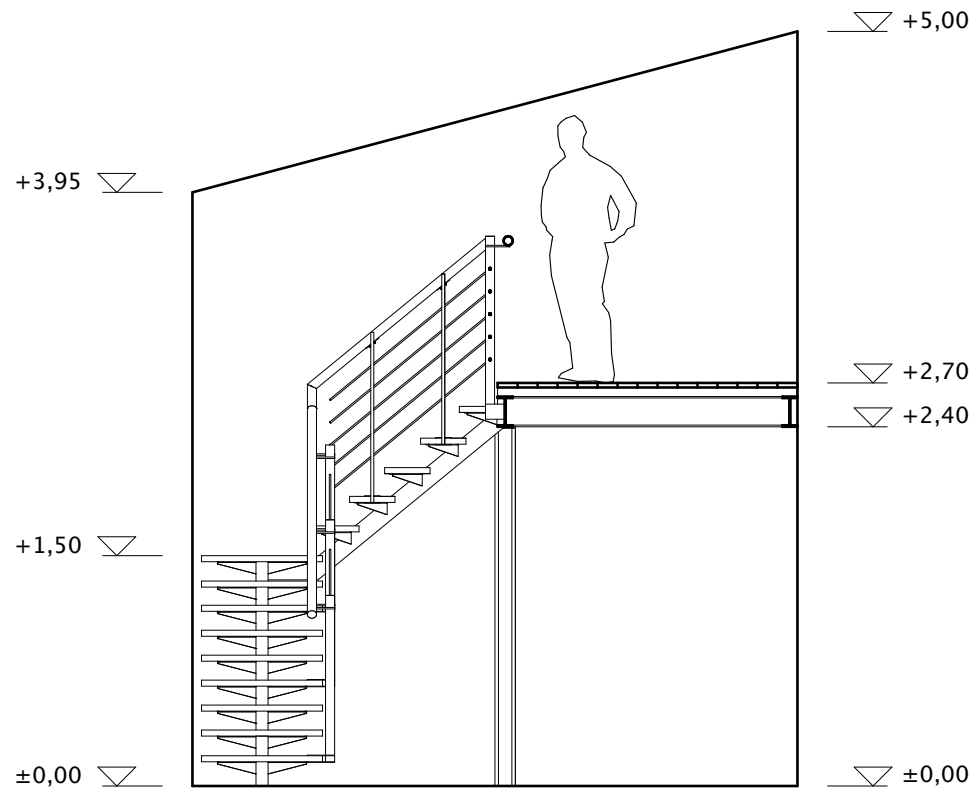
PJŪVIS A-A, M1:50
